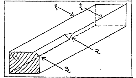
१ Arriis कड. २ Stop chamfer चढता त्रिकोण. ३ Chamfer पाटा.
